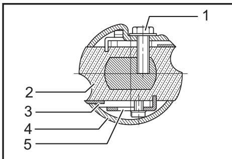
► 1. Pernos 2. Tambor 3. Cuchilla del cepillo 4. Cubierta del tambor 5. Placa de ajuste
